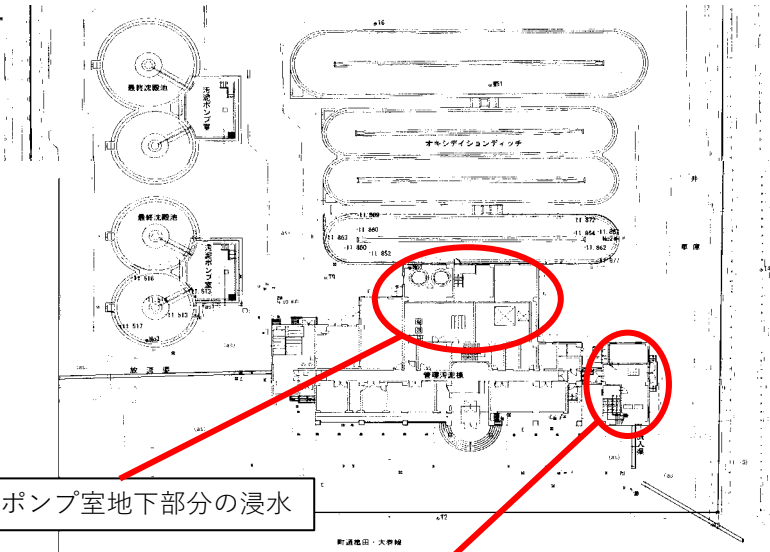
沈砂池・ポンプ棟地下部分の浸水
